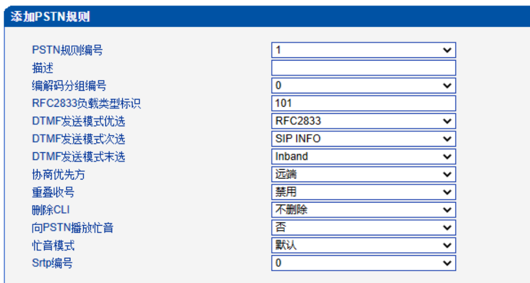
图 2-8-15 添加 PSTN 规则
