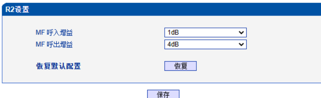
图 2-7-5 R2 设置
